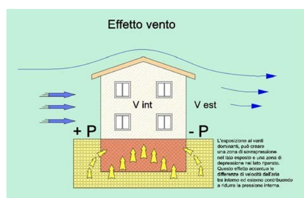
Figura 4: effetto vento
