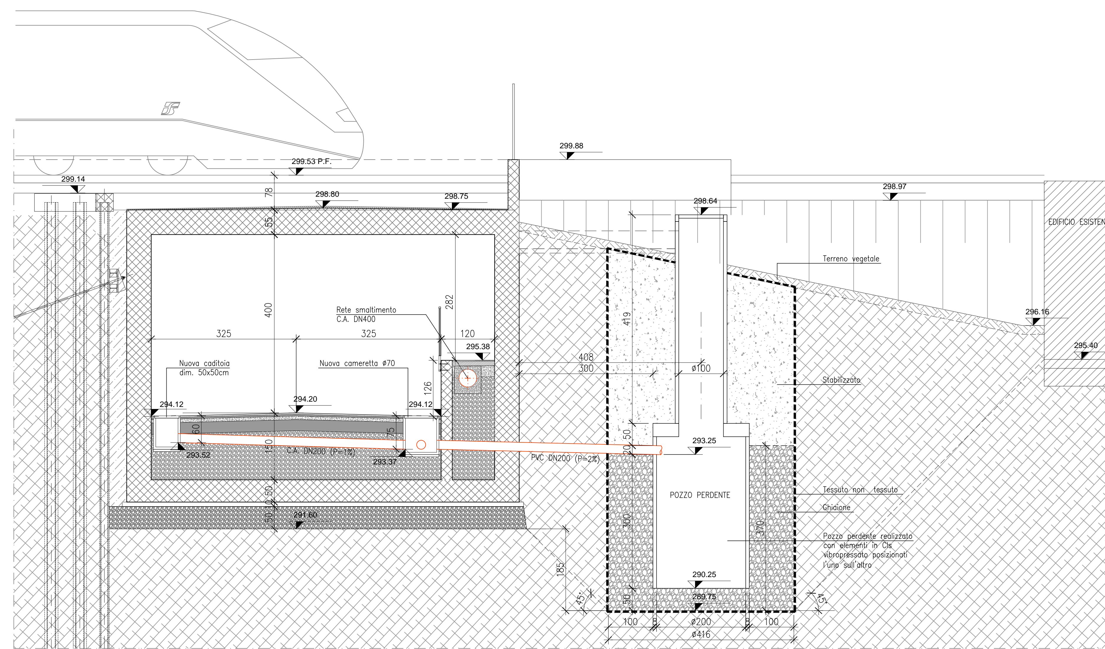
Sezione A-A Scala 1:50
