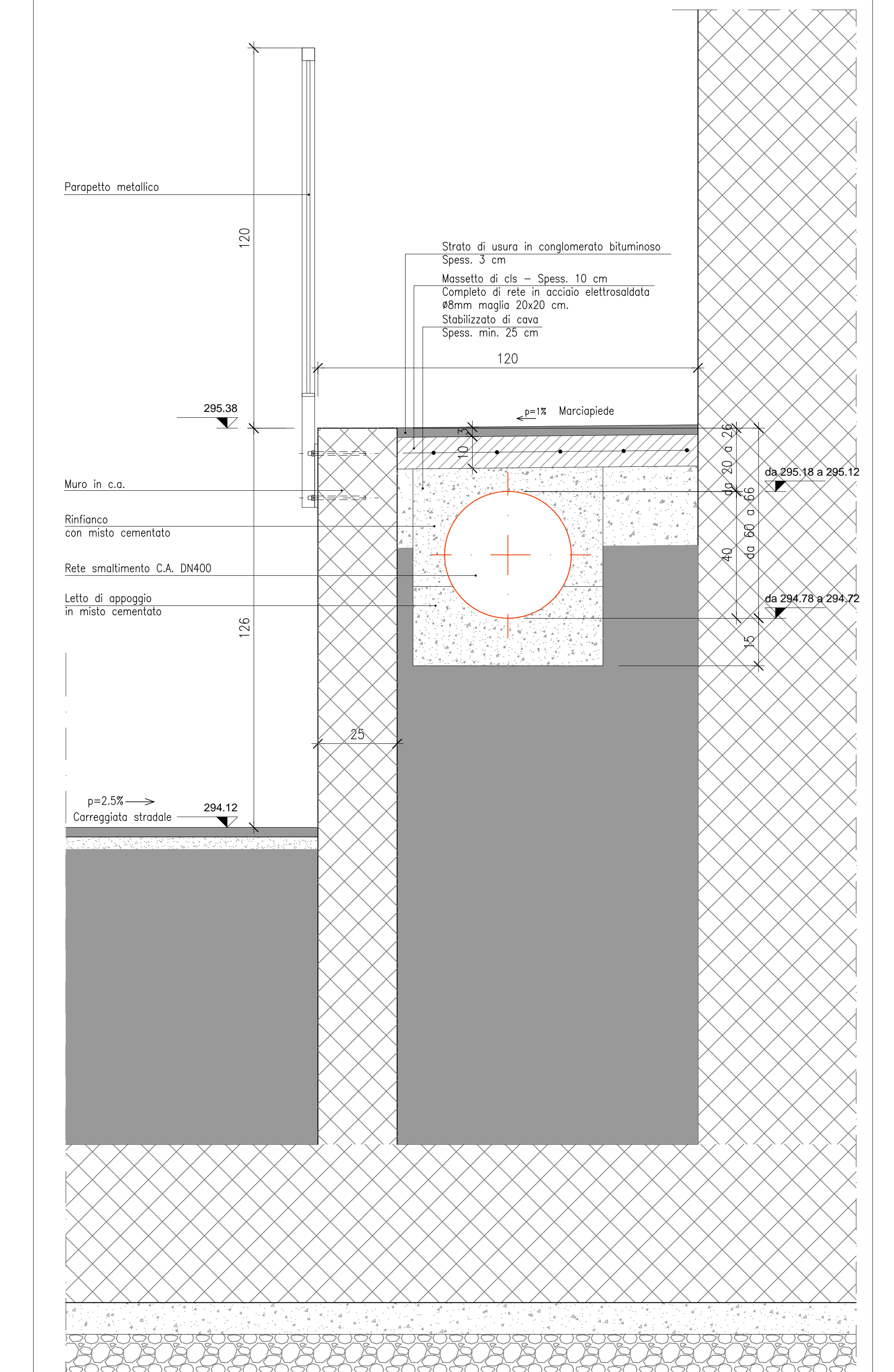
Sezione X-X - Rete di smaltimento Scala 1:10
