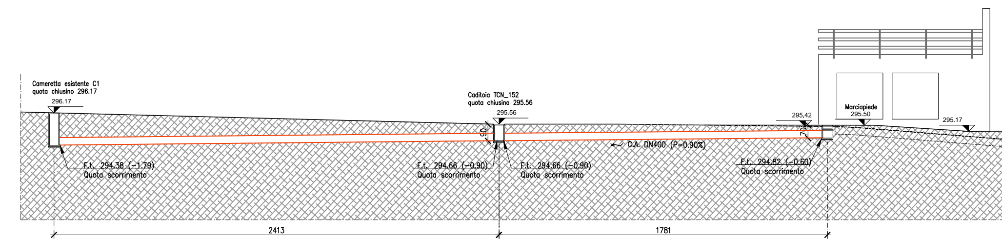
Sezione D-D Scala 1:200
