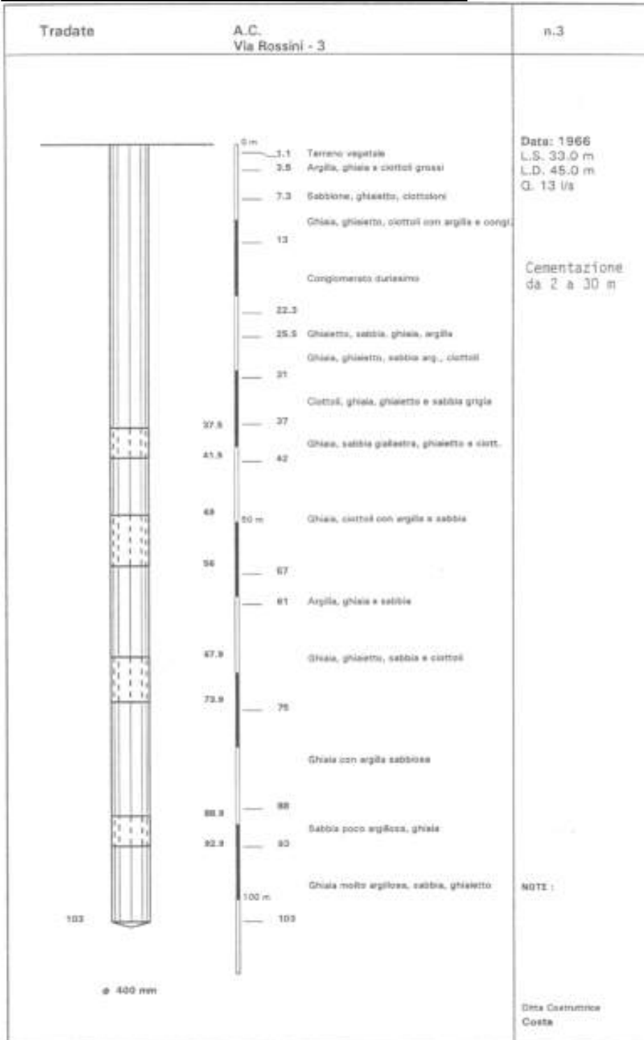
Figura 5: PGT – Stratigrafia Pozzo n°3 di via Rossini
