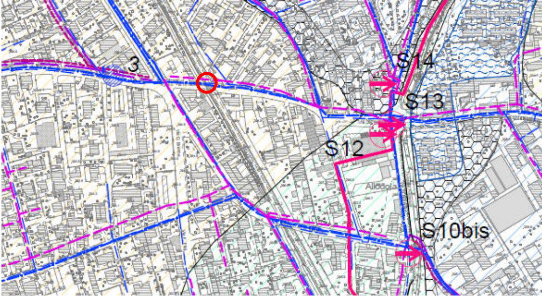
Figura 7: PGT - Carta litotecnica ○ area in esame
