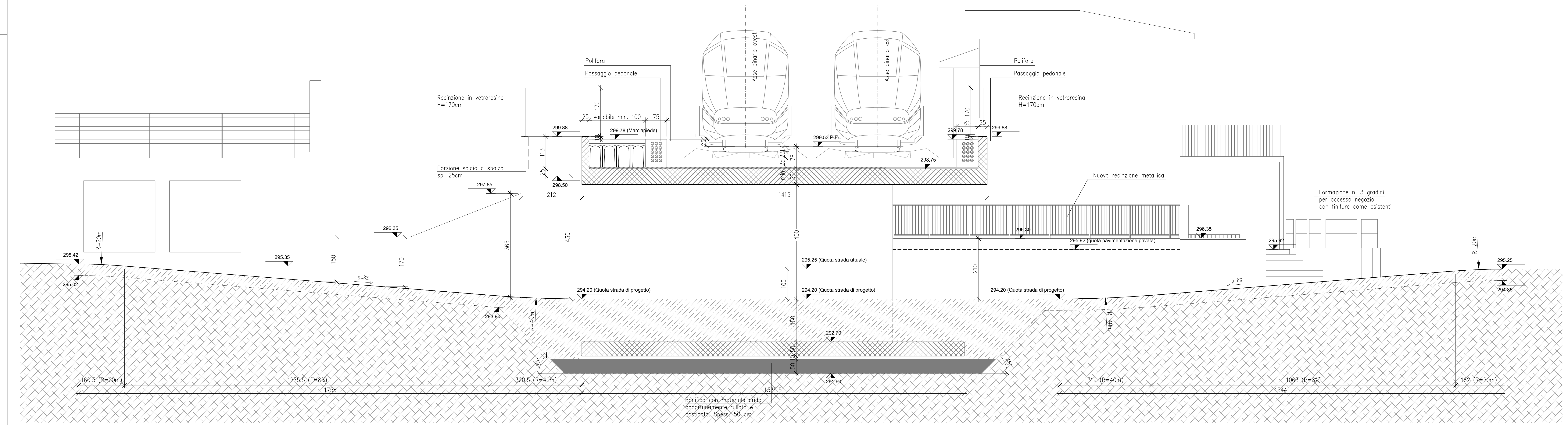
SEZIONE B-B - PROGETTO scala 1:50
