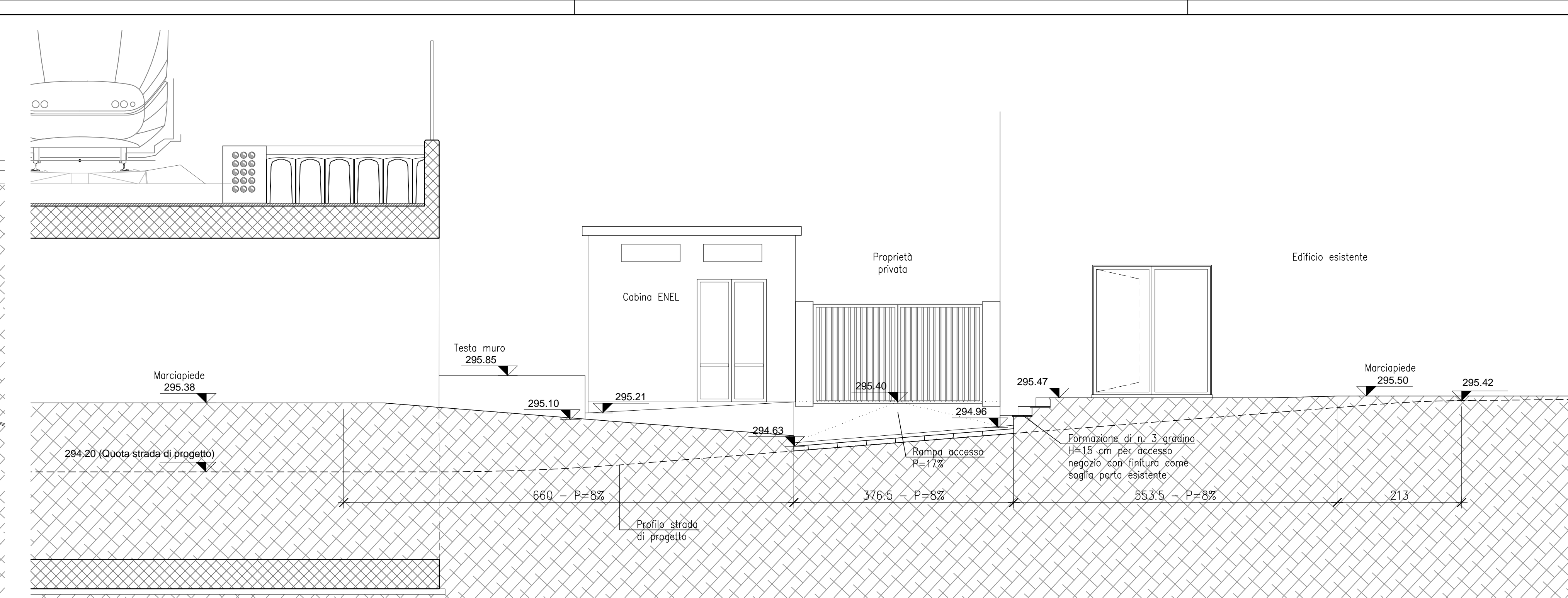
SEZIONE C-C - PROGETTO scala 1:50
