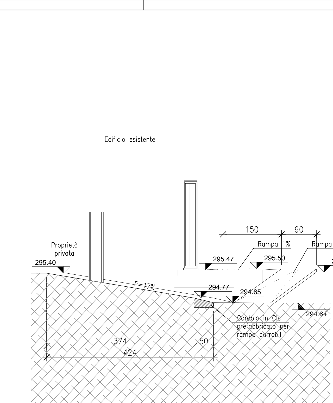
SEZIONE D-D - PROGETTO scala 1:50
