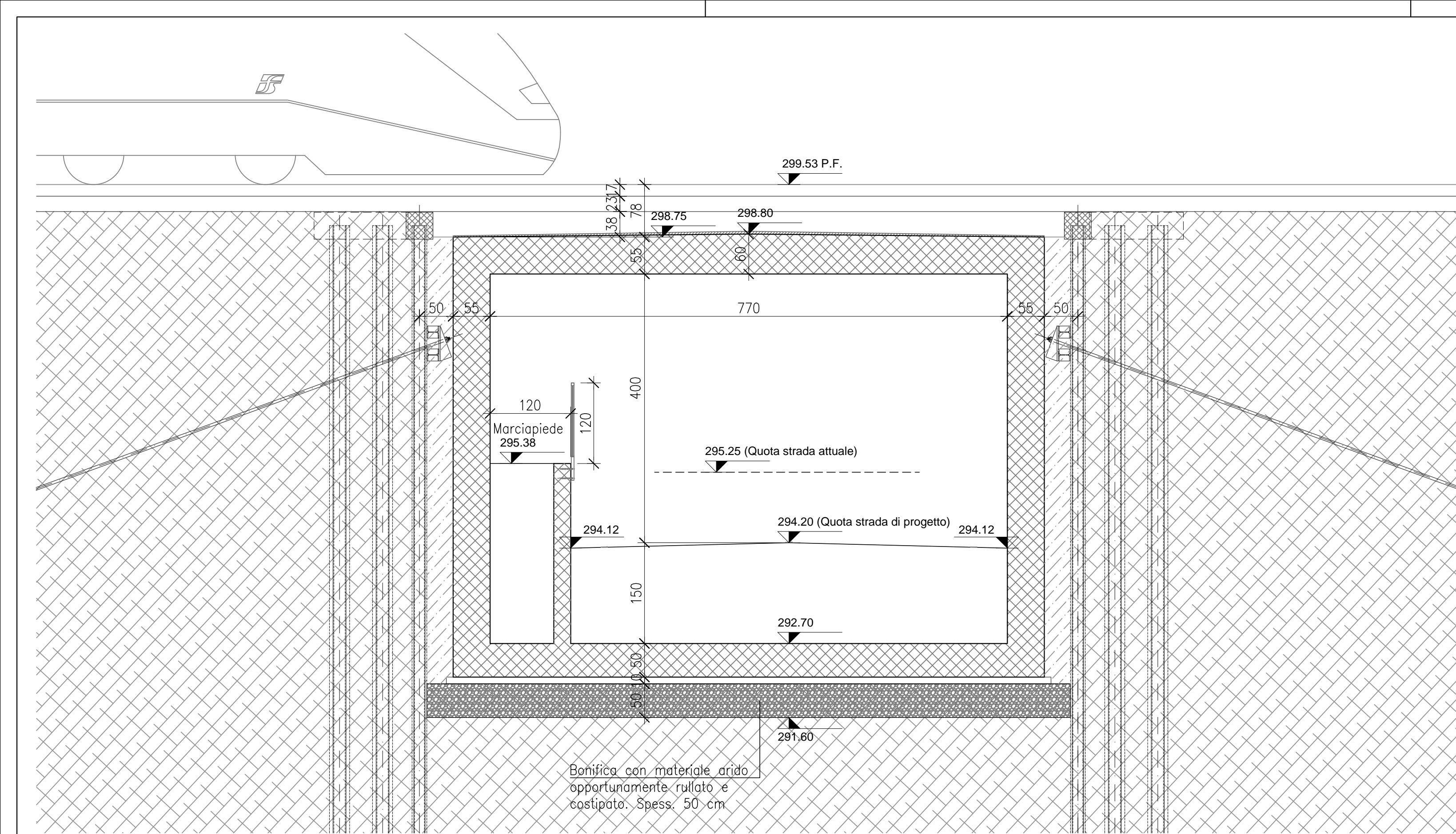
SEZIONE A-A - PROGETTO scala 1:50
