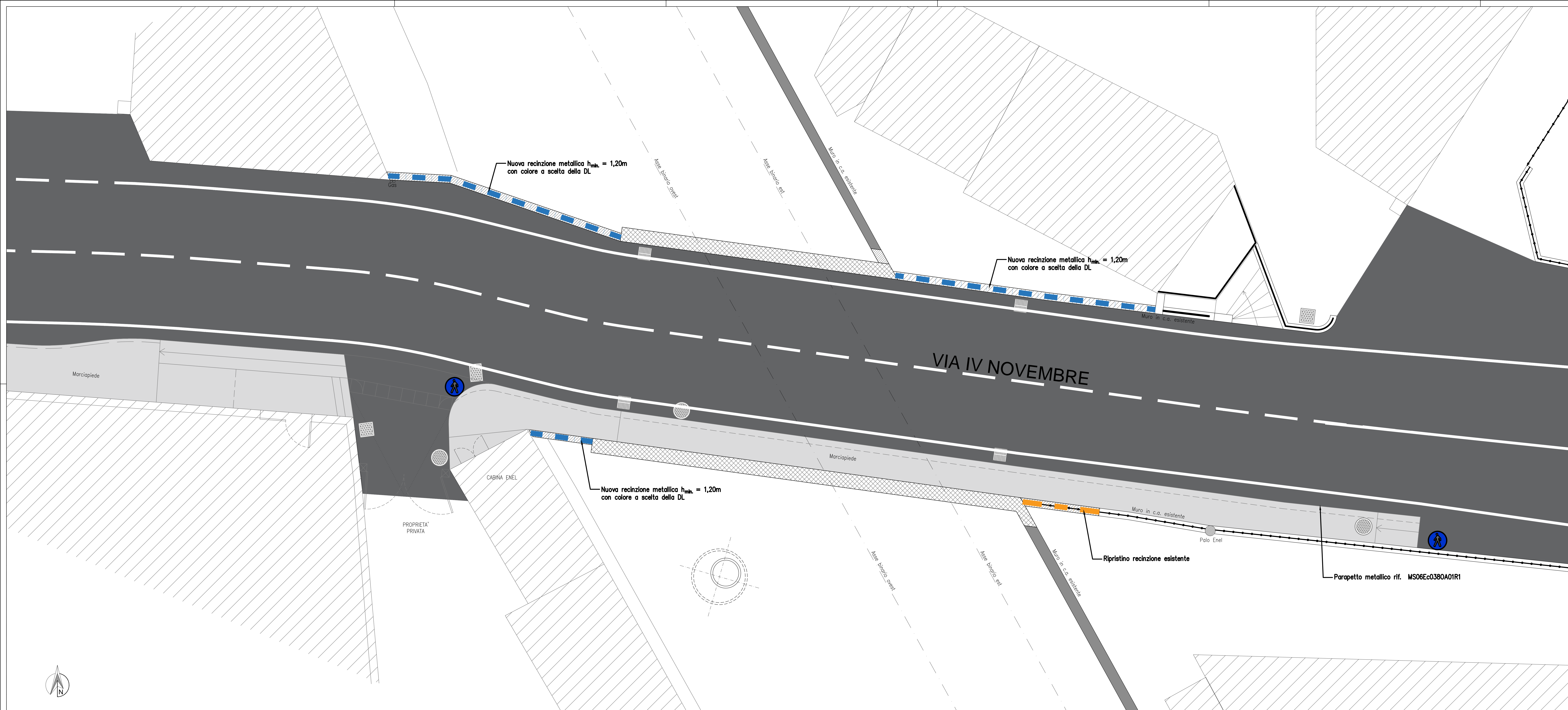
PIANTA PIANO VIABILITA' - PROGETTO scala 1:50
