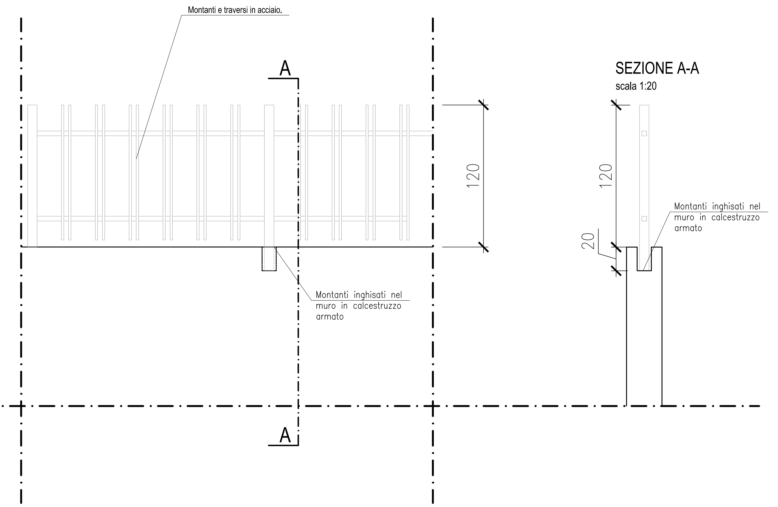
RECINZIONE METALLICA DI CONFINE scala 1:20
