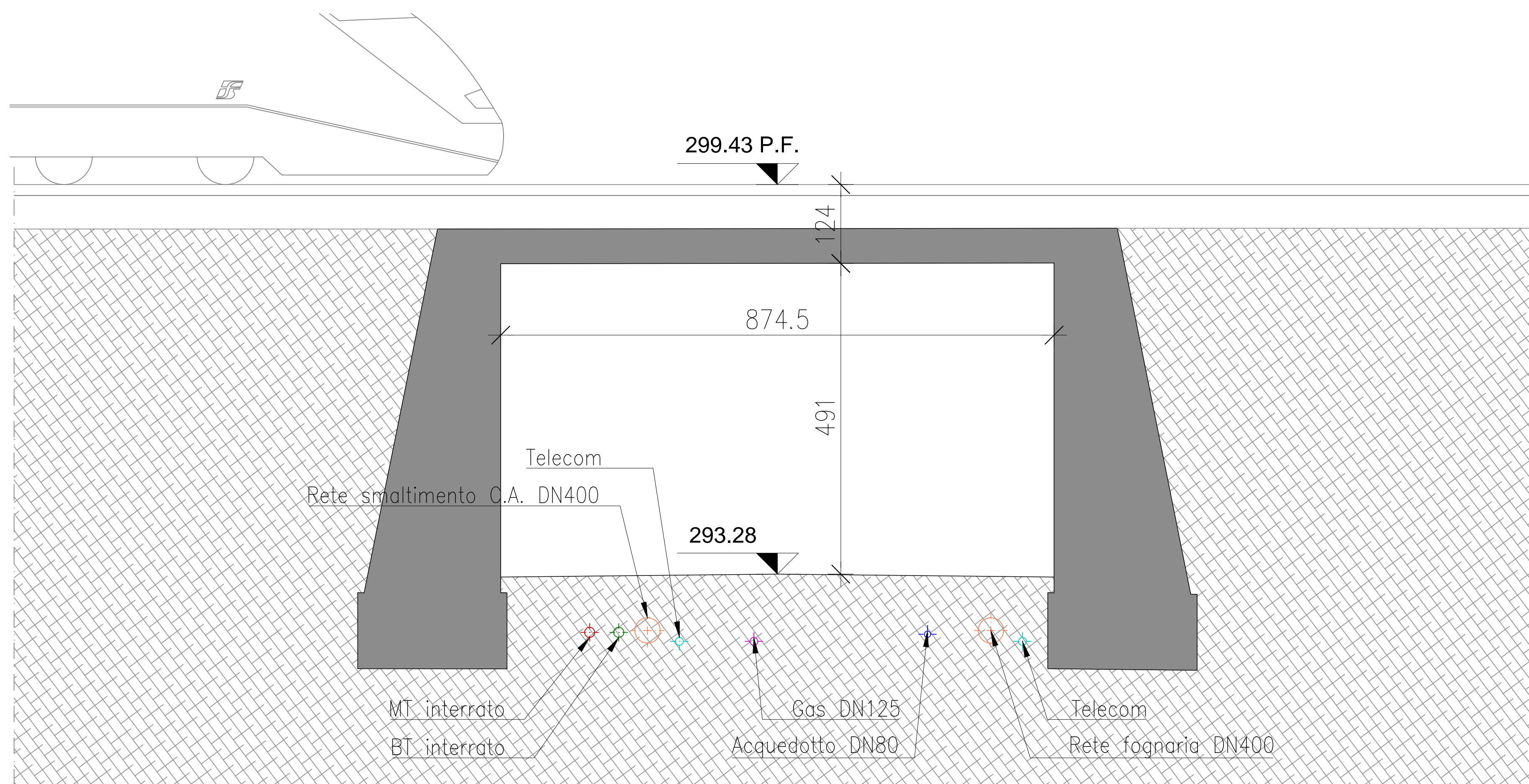
Sezione trasversale - Stato di fatto Scala 1:50
