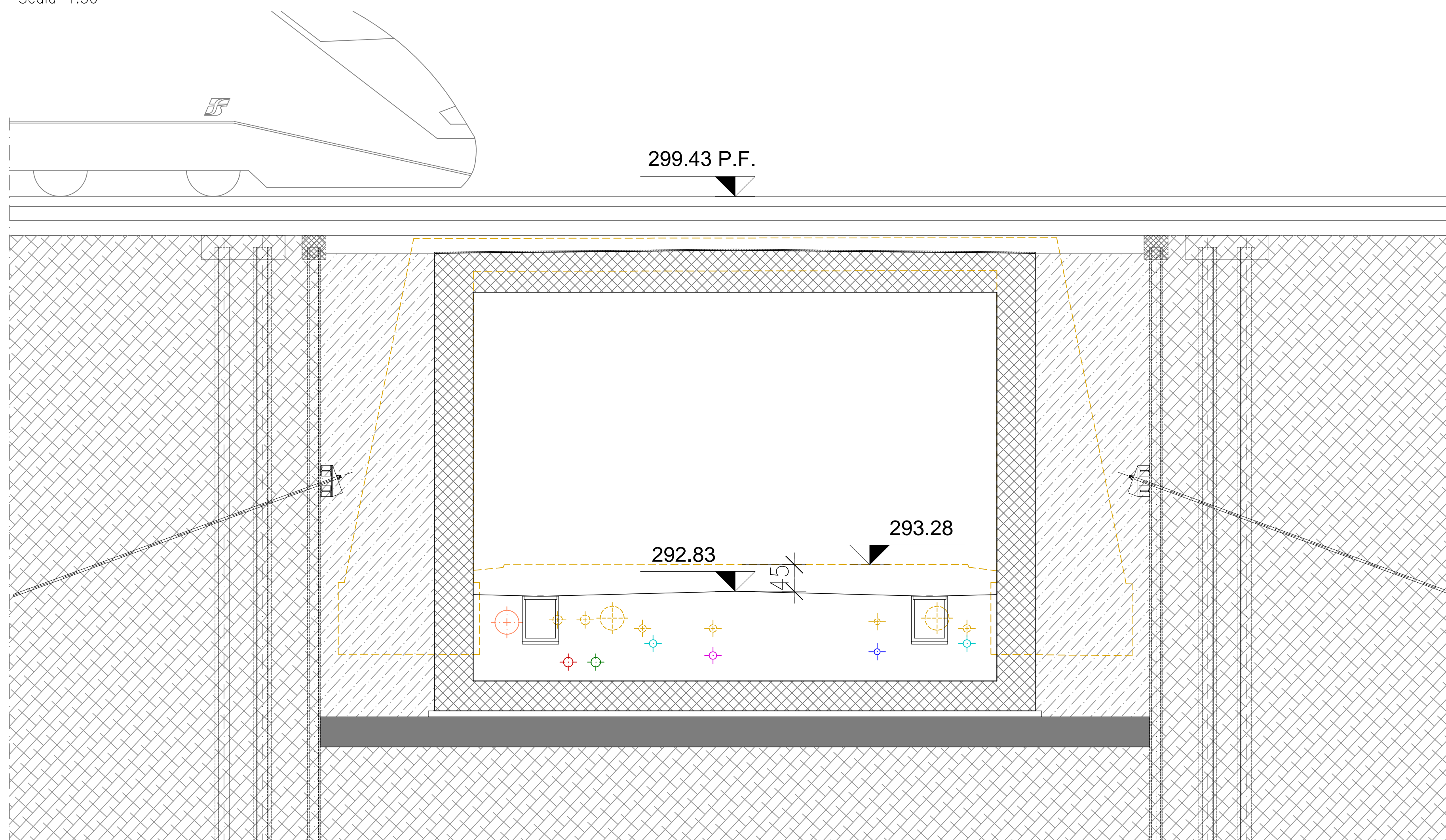
Sezione trasversale - Intervento Scala 1:50
