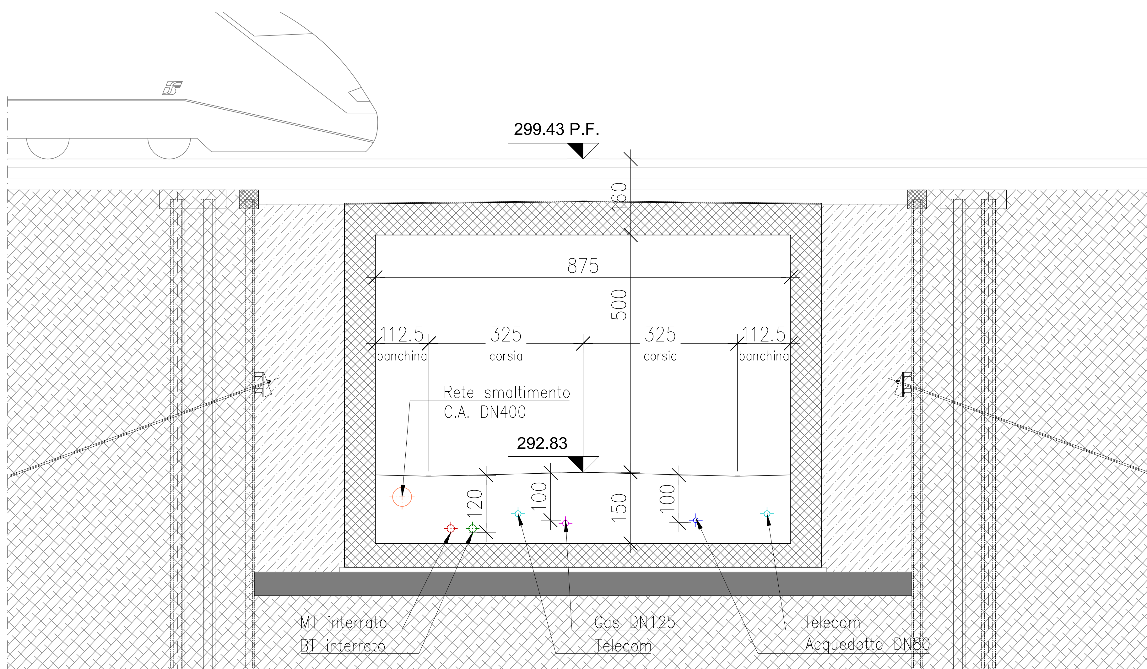
Sezione trasversale - Progetto Scala 1:50
