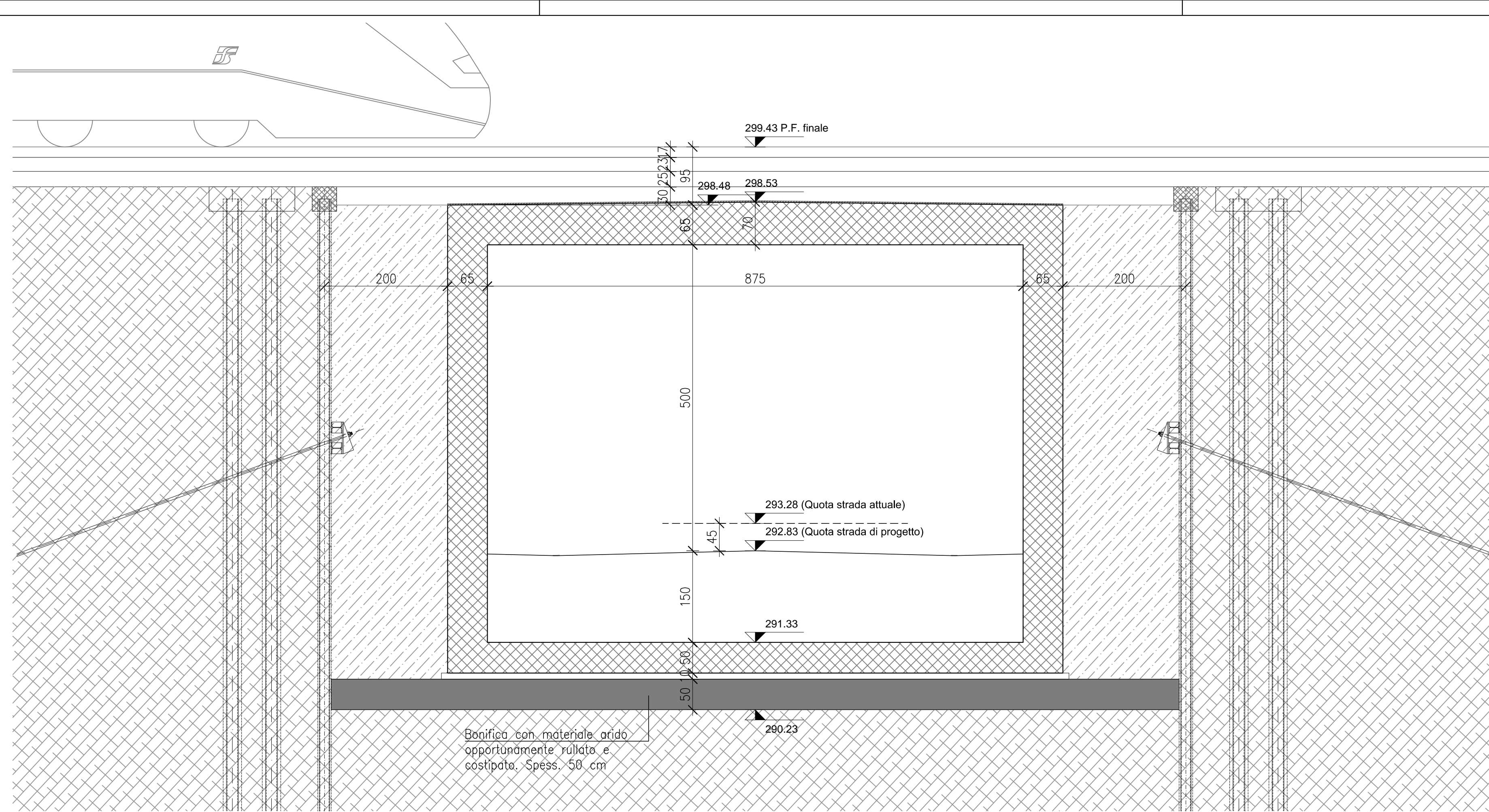
SEZIONE A-A - PROGETTO scala 1:50
