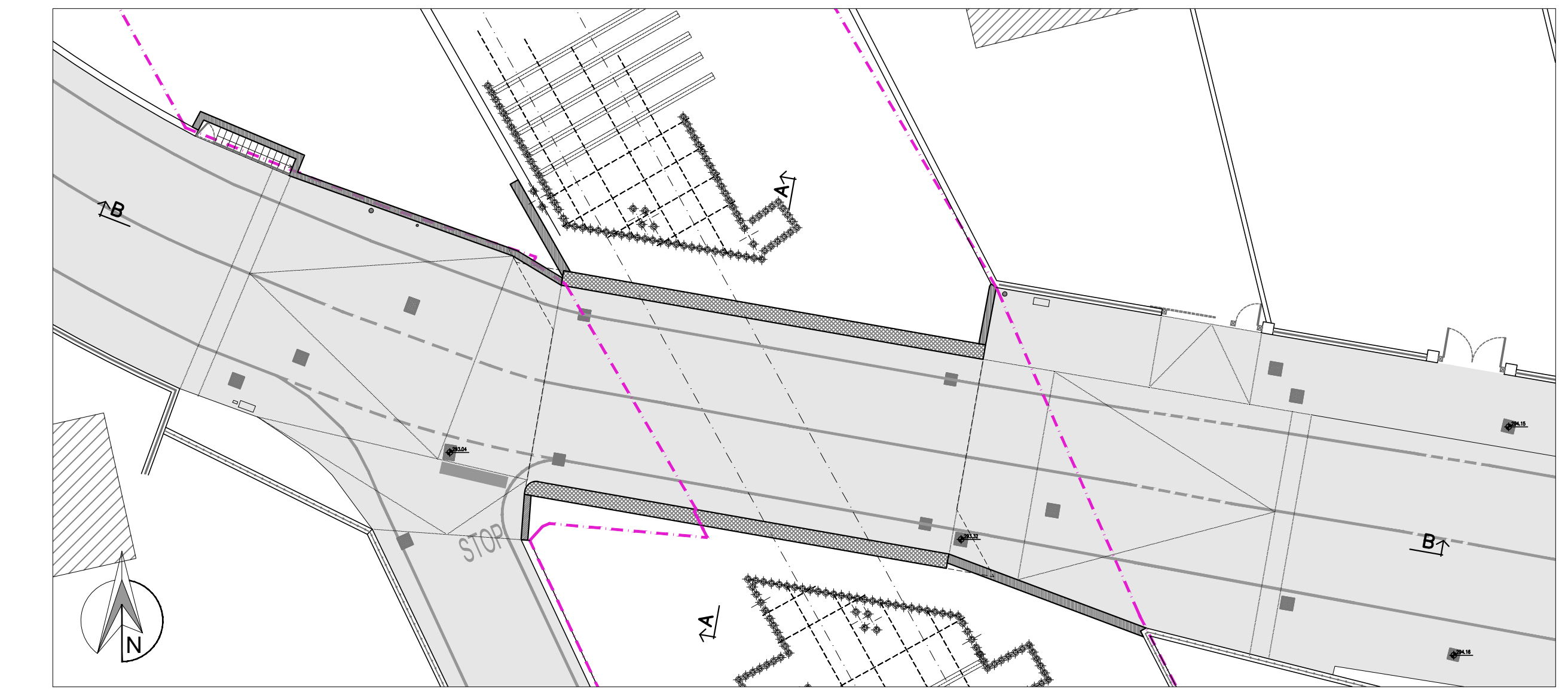
PIANTA CHIAVE scala 1:200
