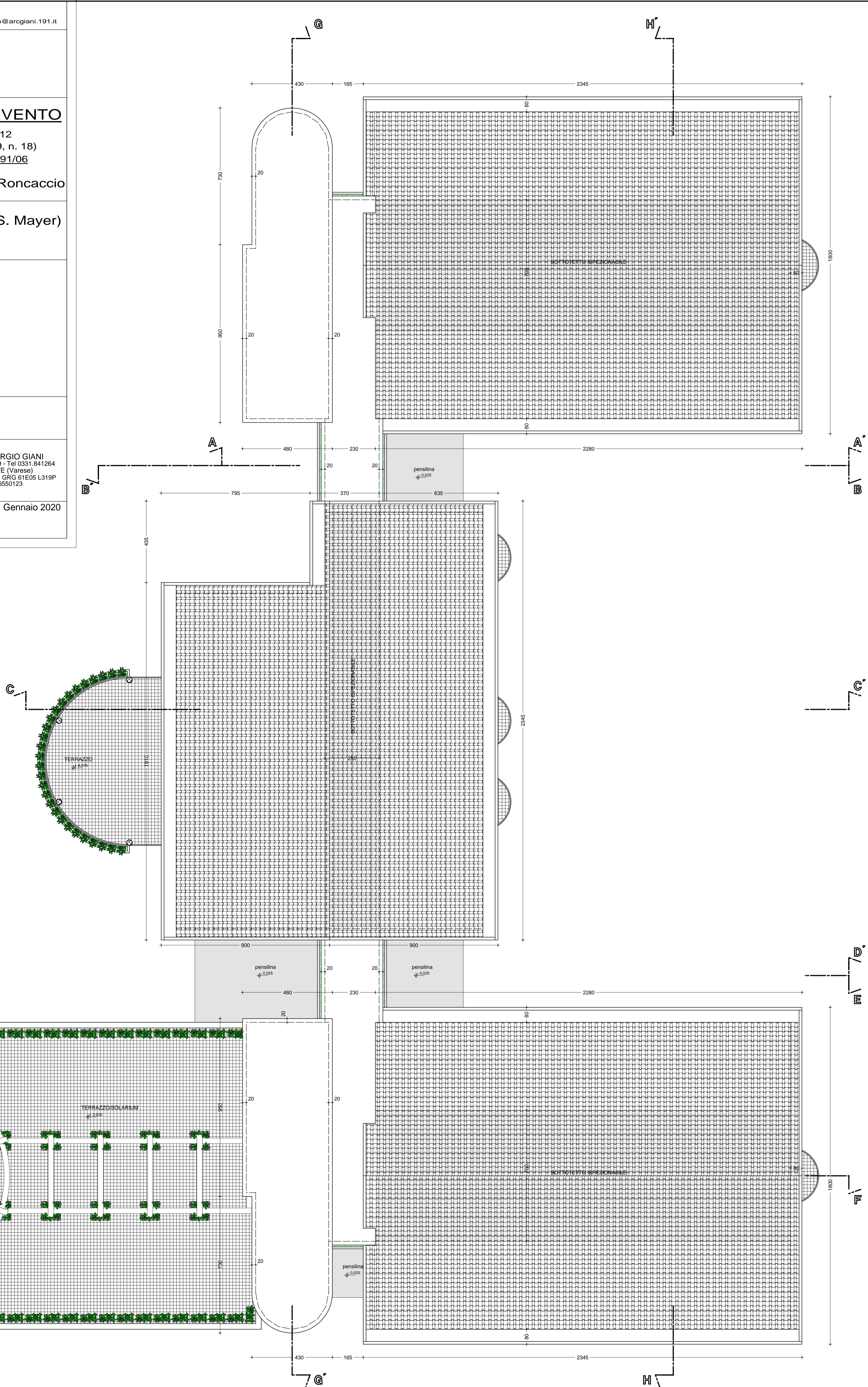
PIANTA COPERTURA
