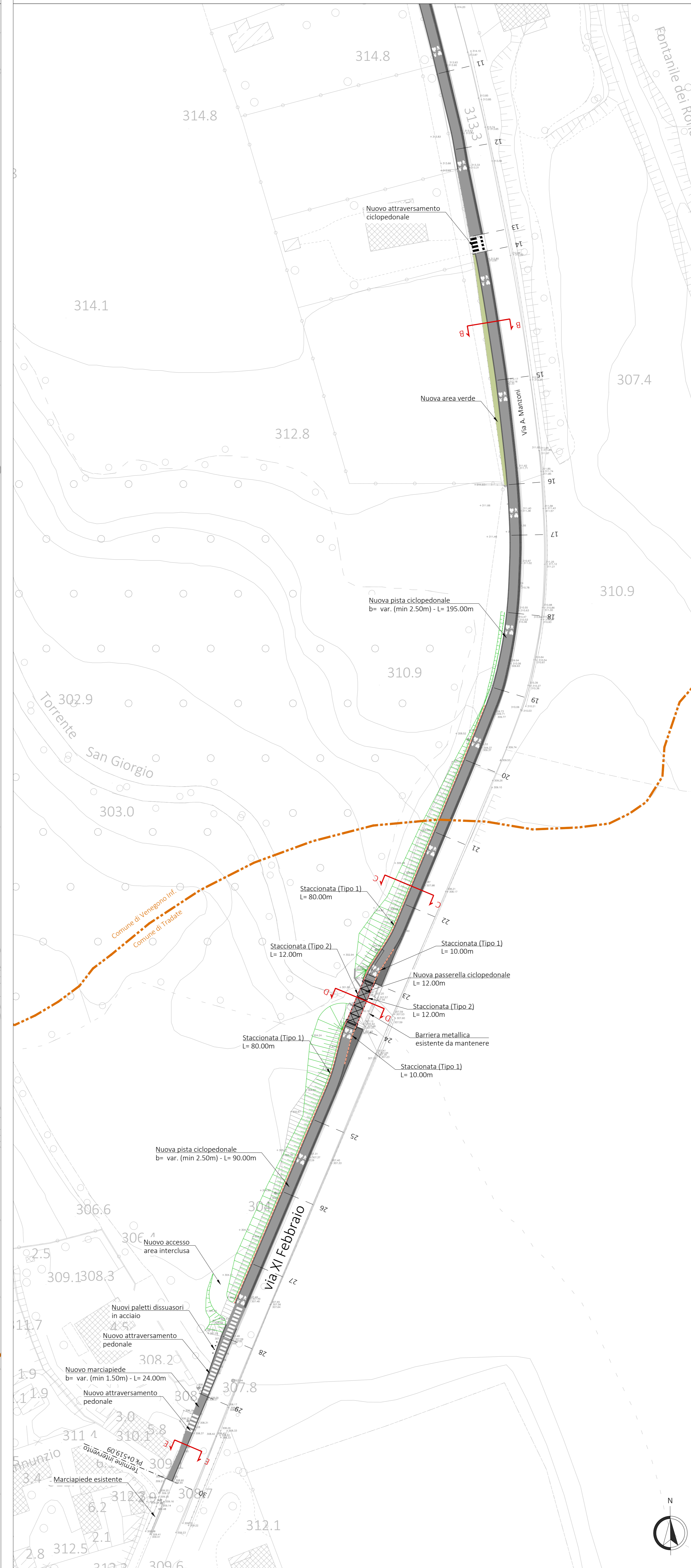
PLANIMETRIA 2° TRATTO - scala 1:500
